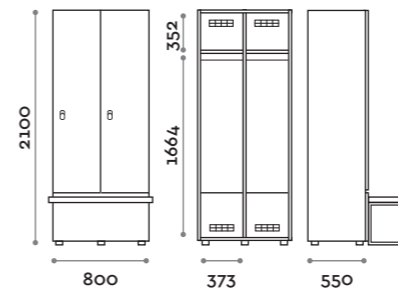
TANB44-23 Doppia colonna 2 ante per panca Double column 1-tier locker, bench- version, full lenght doors
