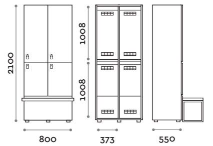
TANB45-23 Doppia colonna 4 ante per panca Double column 2-tiers locker, bench- version, 4 doors
