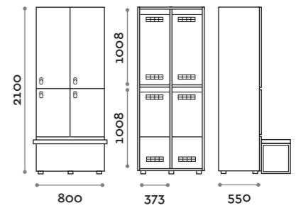
ANB45-23 Doppia colonna 4 ante per panca Double column 2-tiers locker, bench- version, 4 doors
