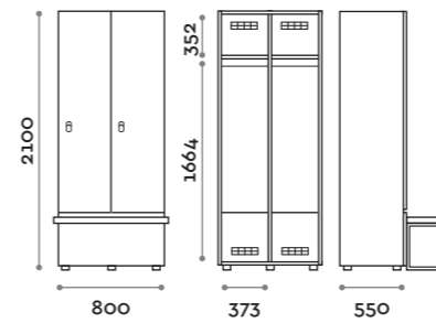
ANB44-23 Doppia colonna 2 ante per panca Double column 1-tier locker, bench- version, full lenght doors
