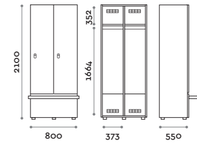
SANB44-23 Doppia colonna 2 ante per panca a sbalzo Double column 1-tierlocker, cantilevered bench version, full lenght doors
